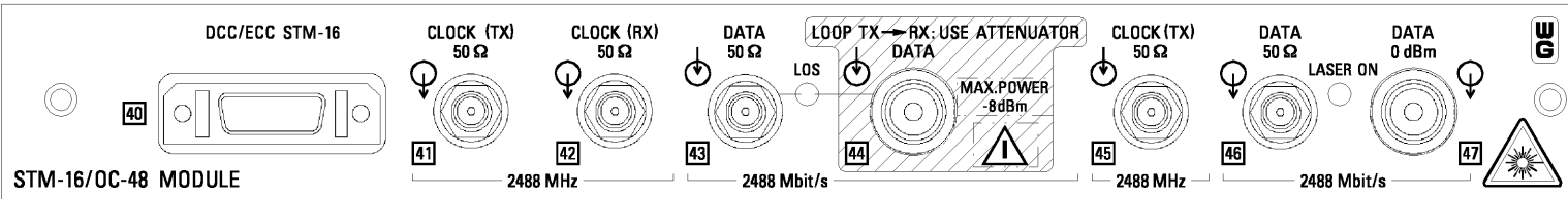
Bild E-1 Anschlußseite des STM-16/OC-48 Moduls
