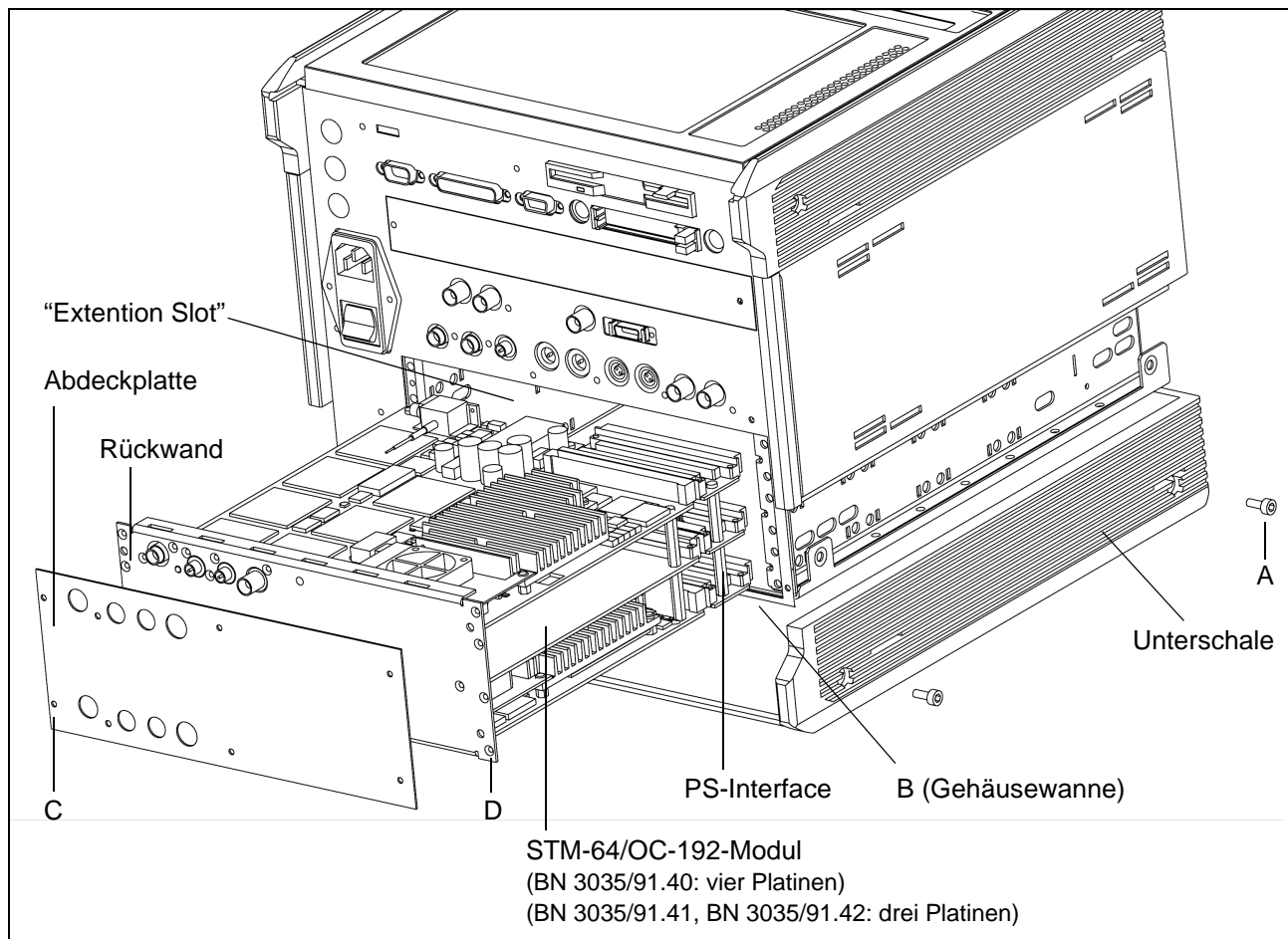
Bild W-5 Einbau der optischen Schnittstelle STM-64/OC-192
