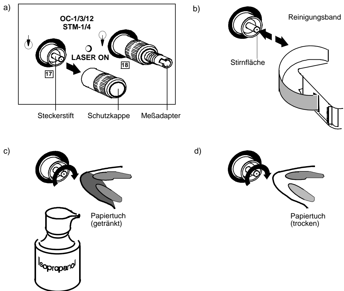
Bild W-2 Meßanschlüsse reinigen
